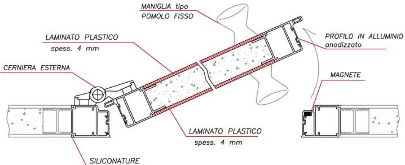
SEZIONE ORIZZONTALE
