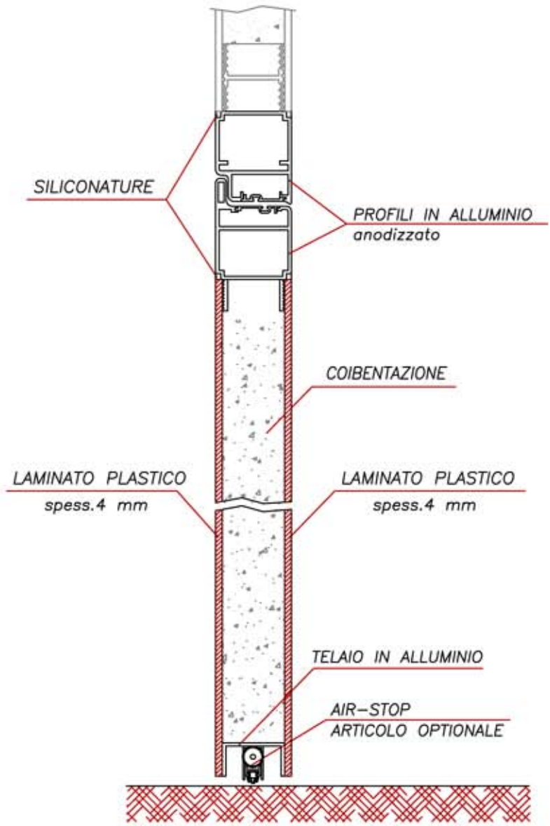
SEZIONE VERTICALE
